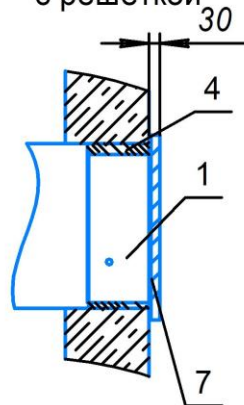
НО(С) установка в преграде до высокого фланца с решеткой
