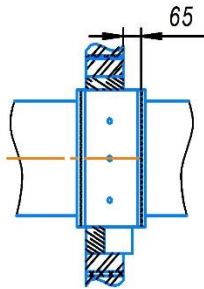
90-НО(КЛ)-СН установка в преграде
