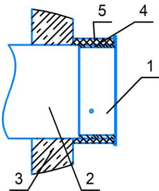
НО(С) установка вне преграды в воздуховоде до высокого фланца
