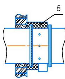
60-НО(КЛ)-СН установка вне преграды
