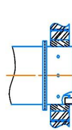
60-НО(КЛ)-ВН установка в преграде
