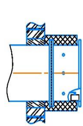
60-НО(КЛ)-ВН установка вне преграды
