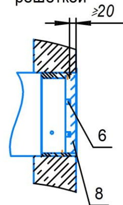
НО(С)-...(БФСУ) установка в глубине преграды с плоской решеткой
