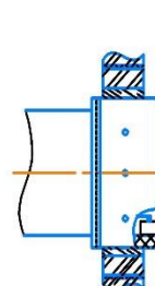
90-НО(КЛ)-ВН установка в преграде
