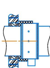
90-НО(КЛ)-СН установка вне преграды
