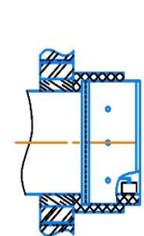
90-НО(КЛ)-ВН установка вне преграды
