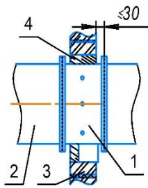
90-НО(КЛ)-СН установка в преграде
